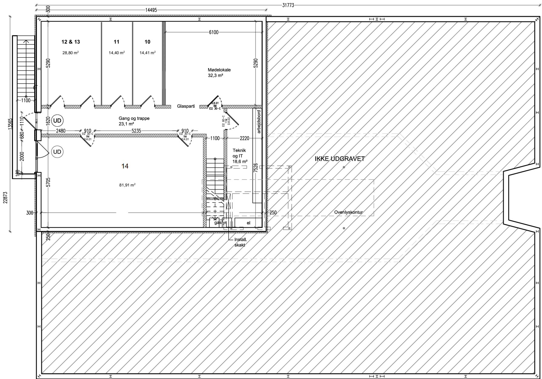
Kælderplan 200,0 m²
