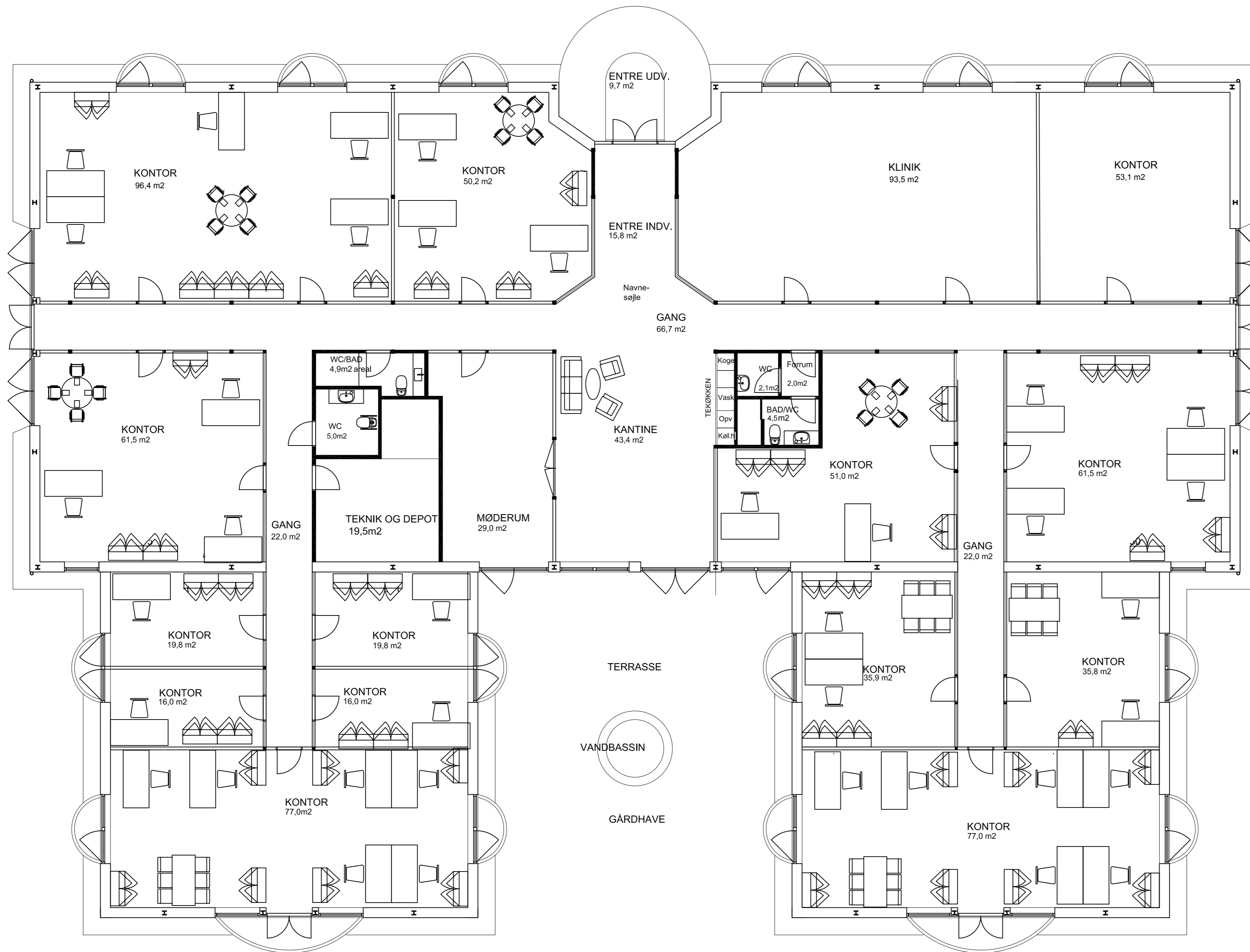
STUEPLAN 1028,4 m 2
