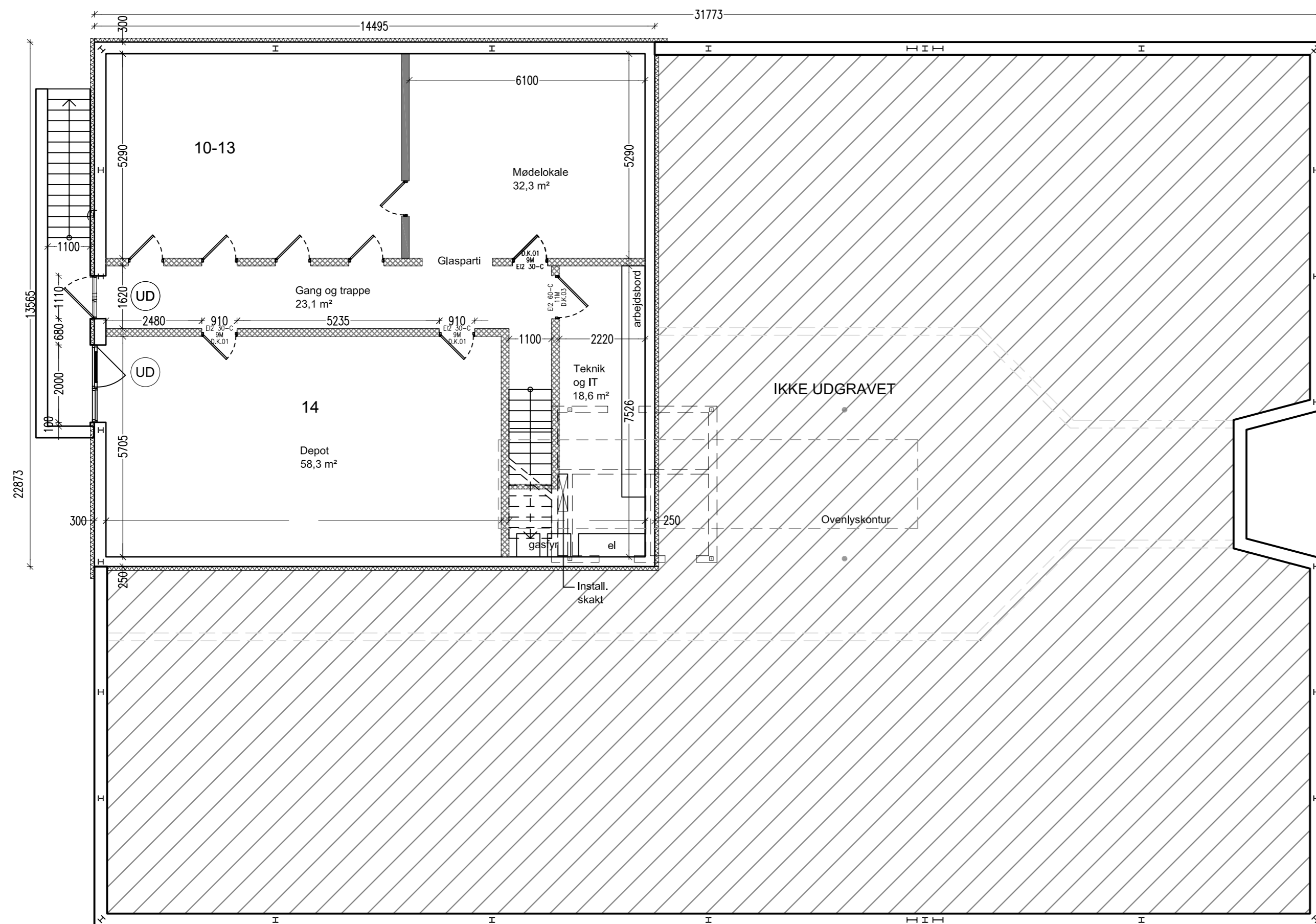
Kælderplan 200,0 m 2
